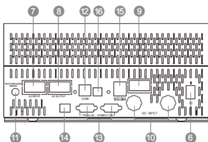
Модель 3кВт – 5,5кВт при параллельном подключении
